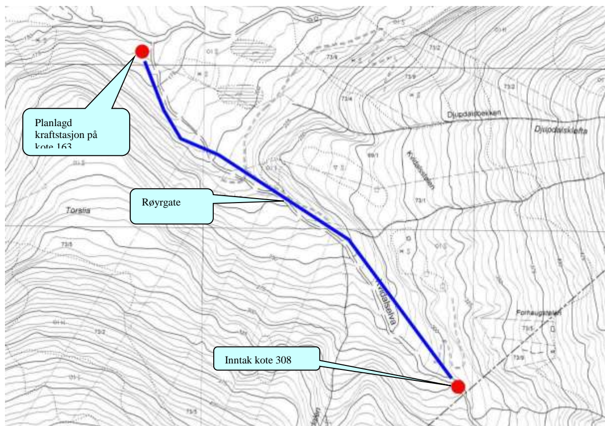
Figur 3. Kartutsnittet viser i grove trekk dei viktigaste naturinngrepa i form av inntak, tunnelar, røyrgater og kraftstasjon.
